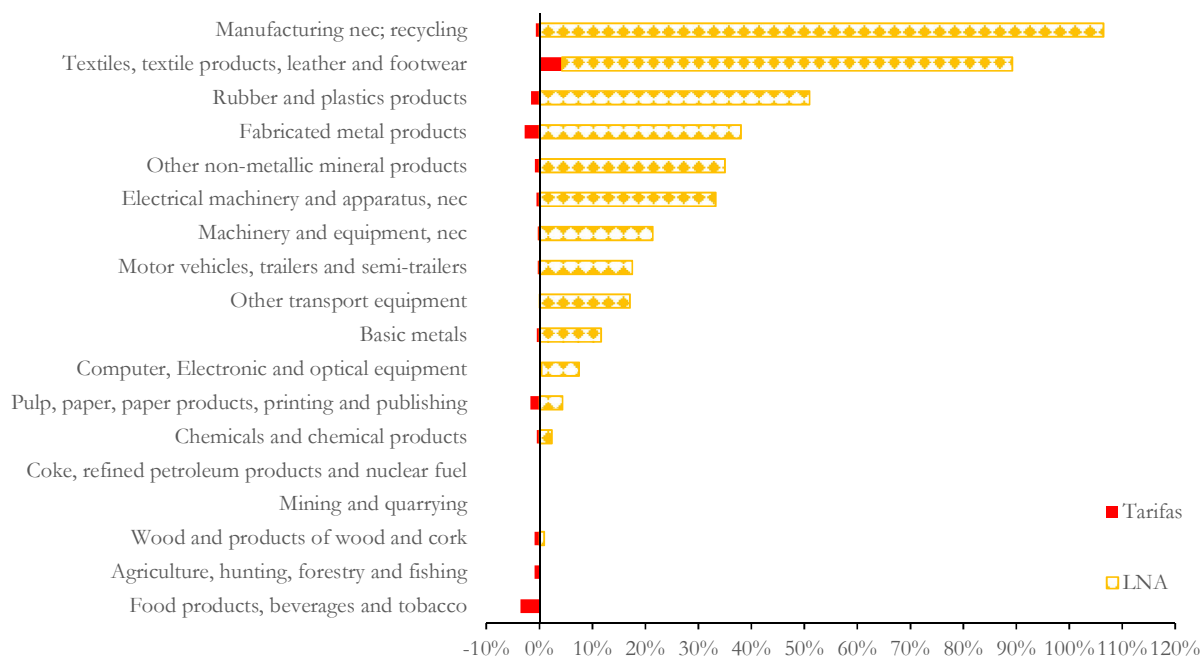
Gráfico 15. Fuente de los cambios en los precios de consumidor de bienes importados según sector productor
